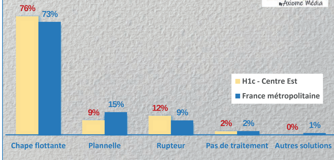
Le traitement thermique du RDC en cas d'isolation par l'intérieur
